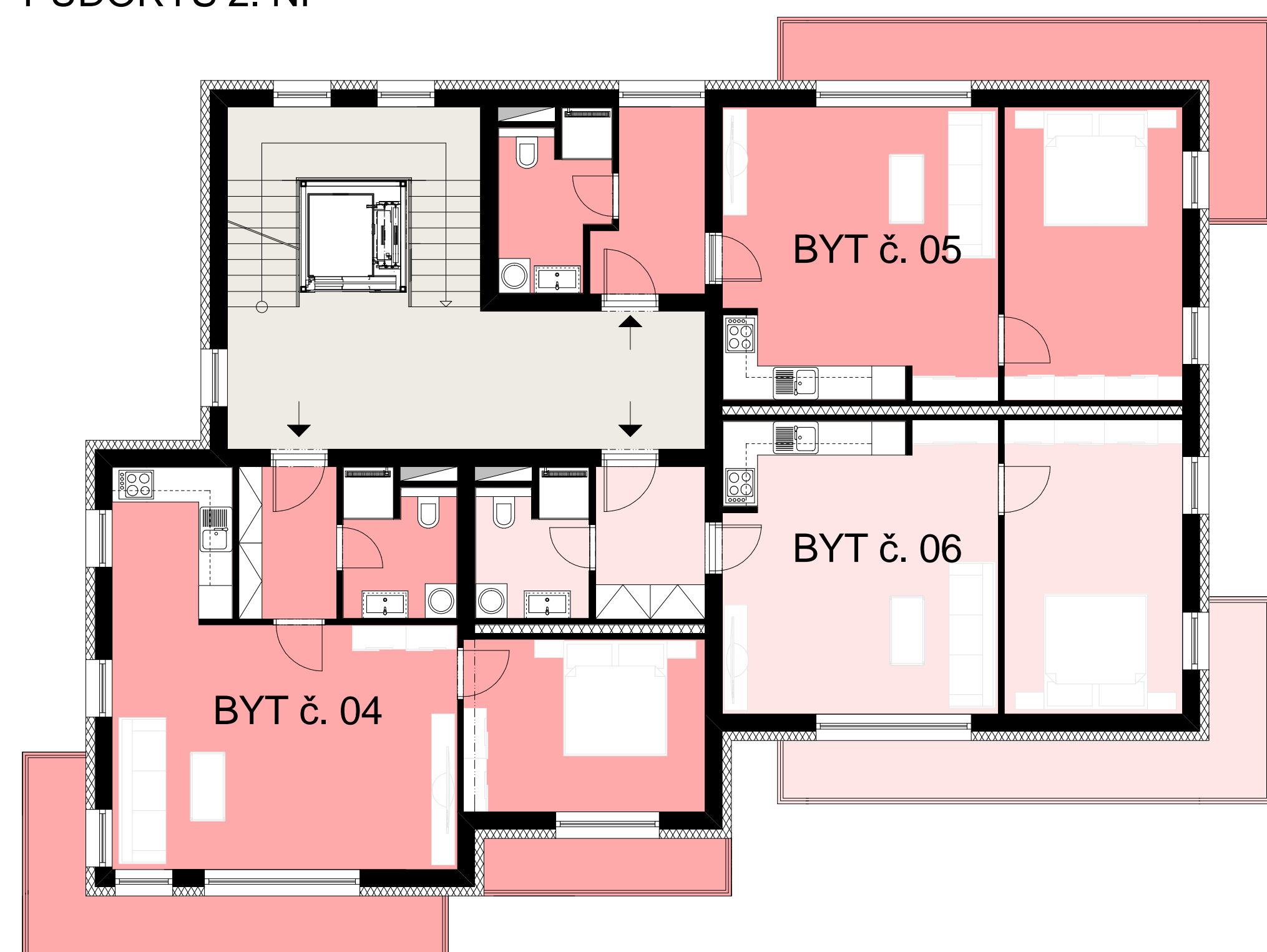
PŮDORYS 2. NP
