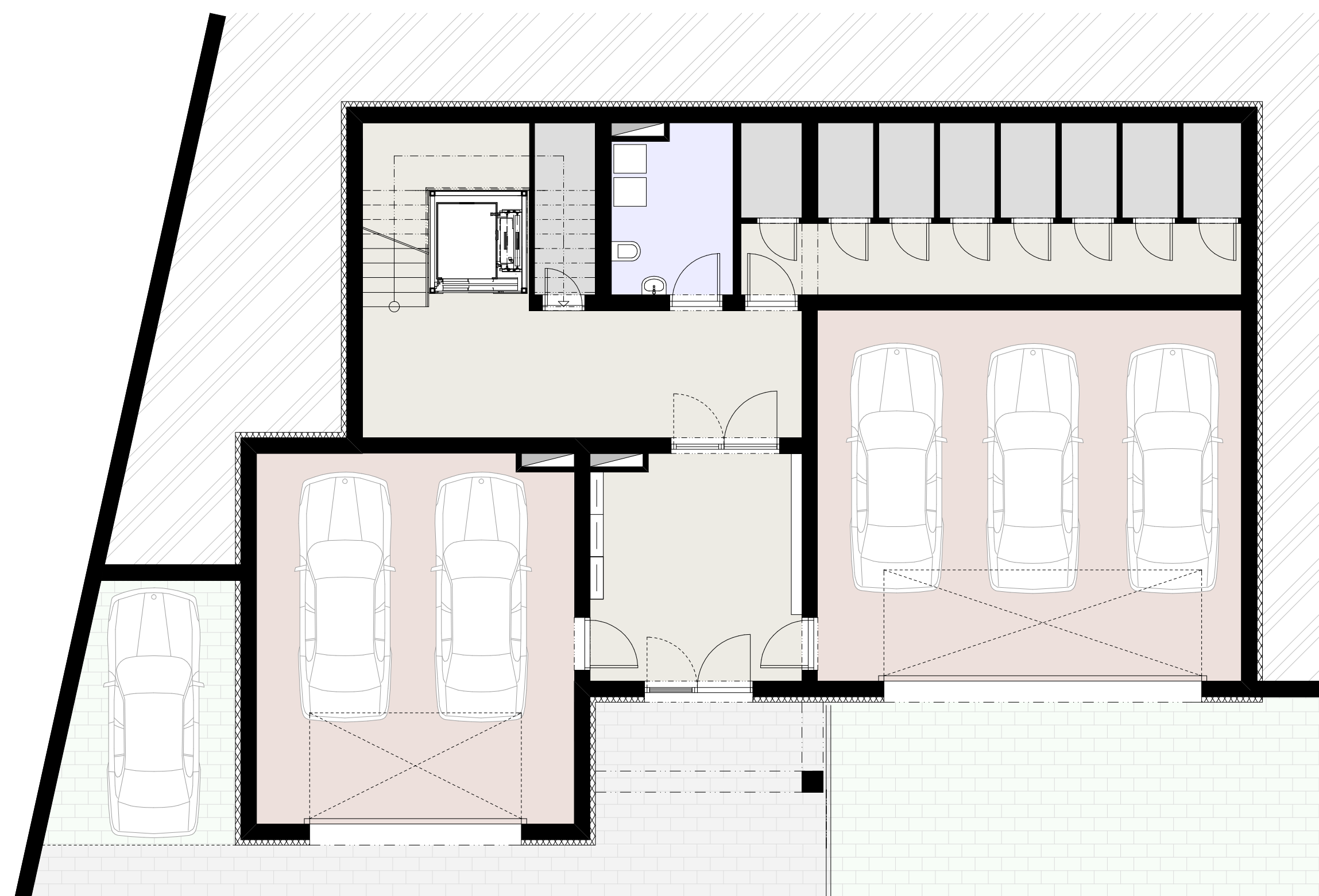
PŮDORYS 1. PP
