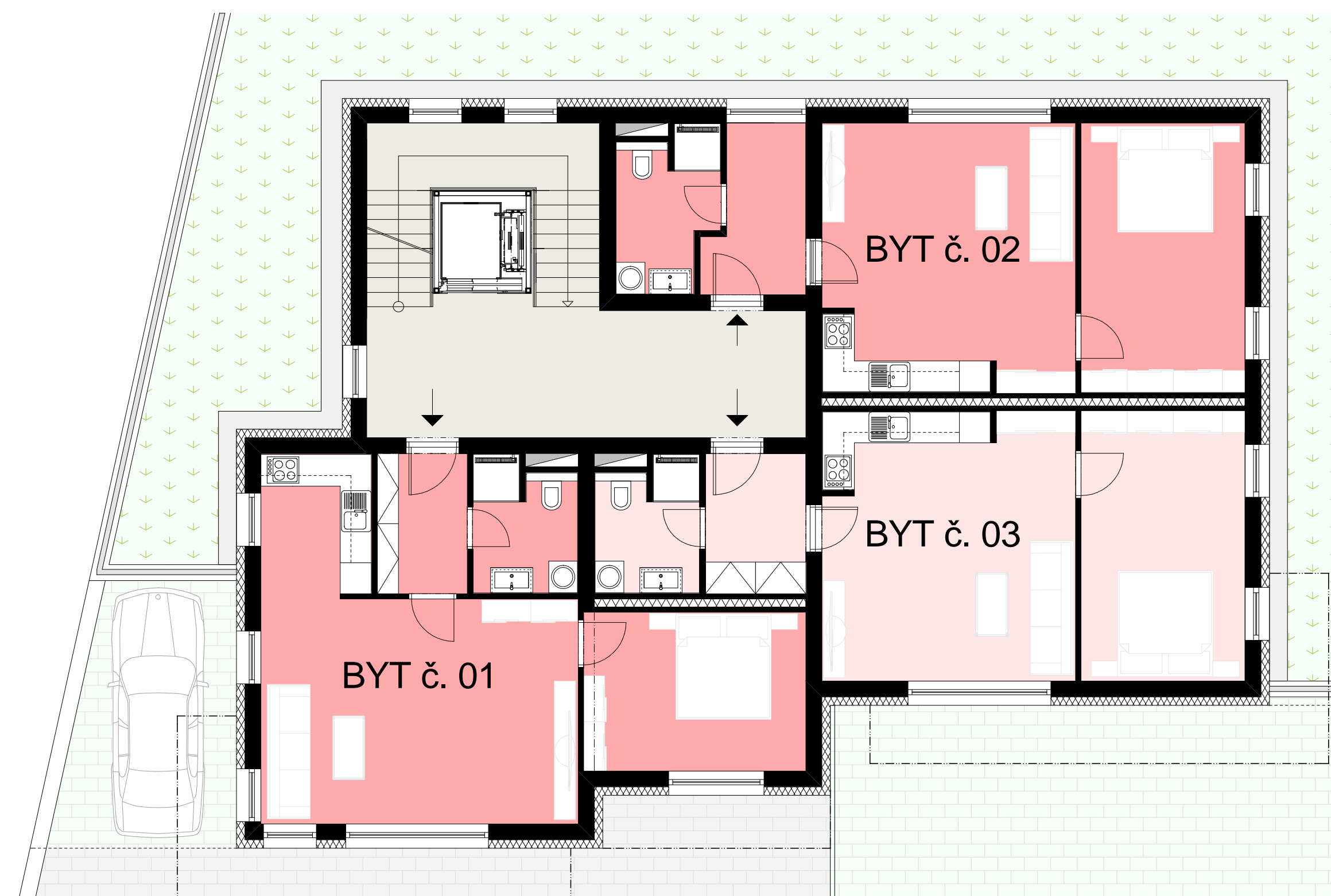
PŮDORYS 1. NP
