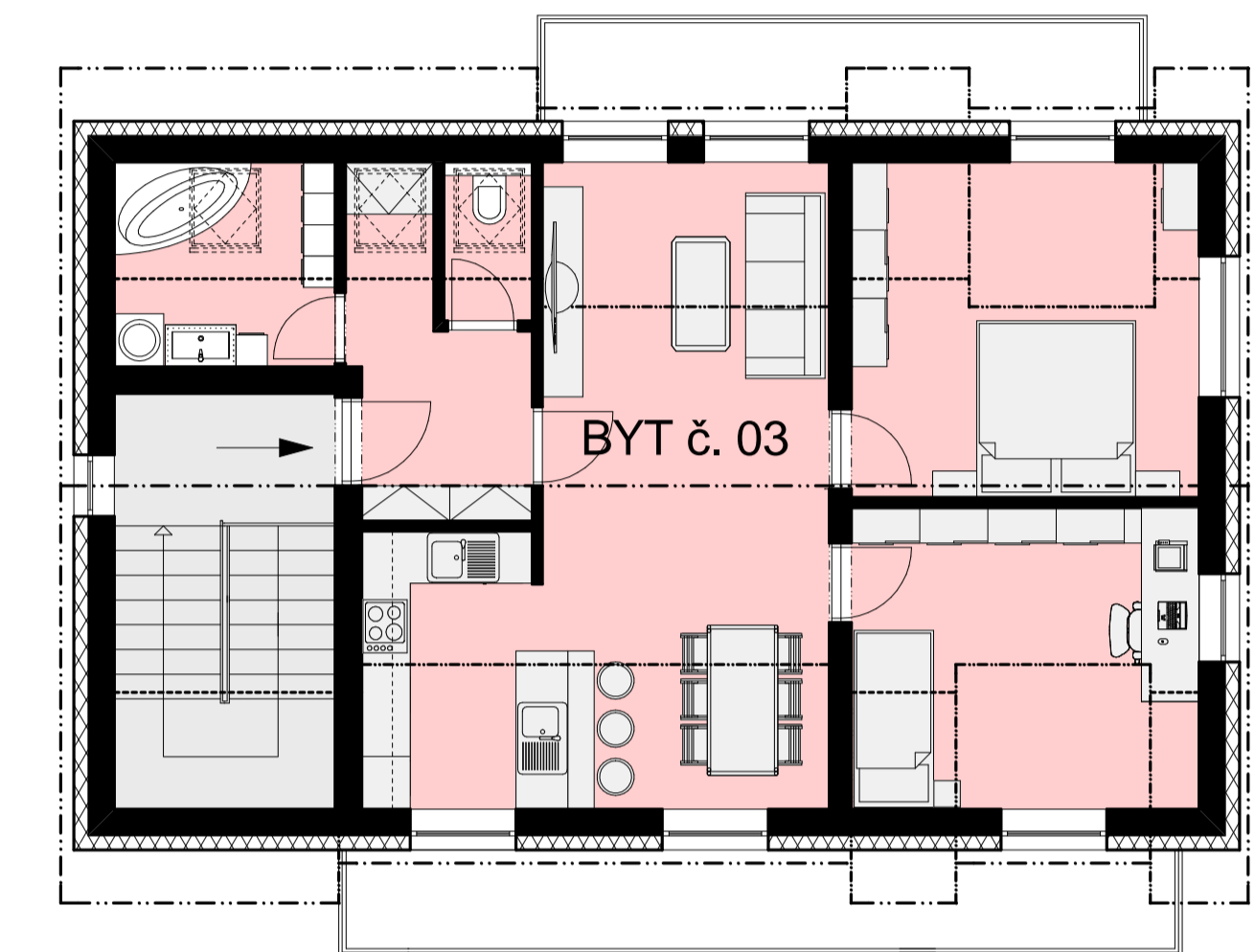
PŮDORYS 3. NP
