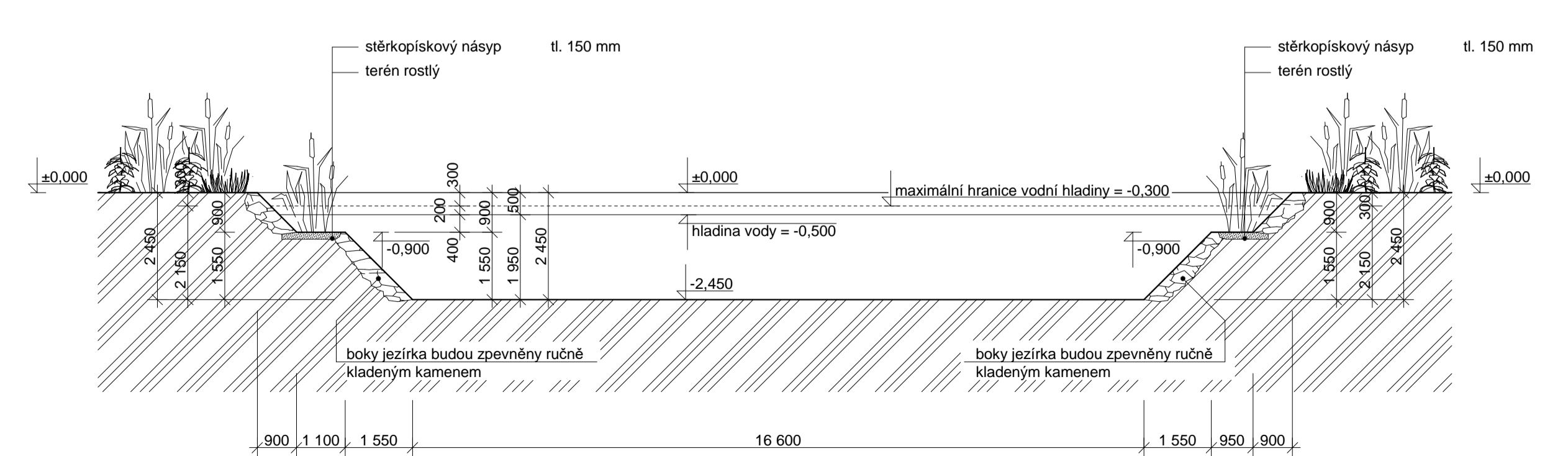
ŘEZ B-B' 1: 100
