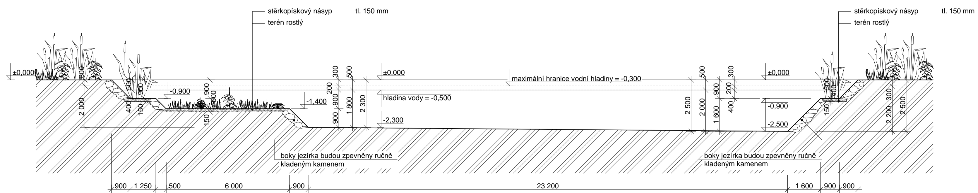
ŘEZ A-A' 1: 100
